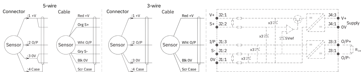
Connector Pin Layout: DIN 43650 C
