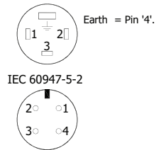
Connector Pin Layout: DIN 43650 C
